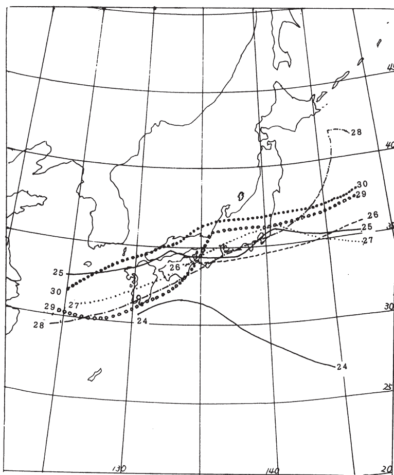
図-2 昭和36年6月24日～30日の梅雨前線の位置 (全国防災協会編『わが国の災害史』より) *毎日9時、数字は日を示す
