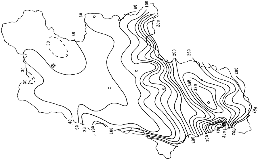
図-10b 長野県下の日雨量分布図
