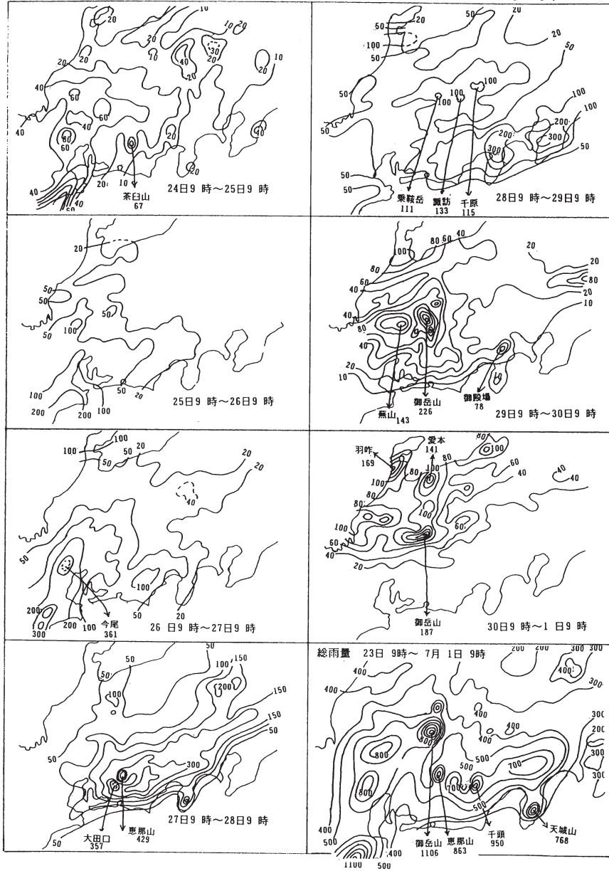
図-9 昭和36年6月24日～7月1日の中部地方の日雨量分布図 および6月23日9時～7月1日の総雨量分布図 (東京管区気象台『異常気象報告』第2巻第2号より)
