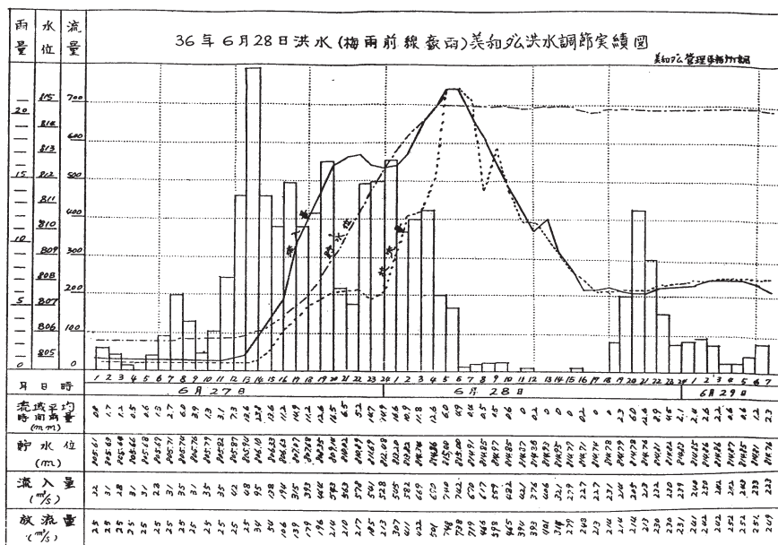
図Ⅱ-8 美和ダム洪水調節実績図
