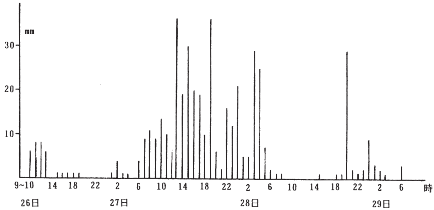
図-11 昭和36年6月26日～29日の飯田における1時間降水量
